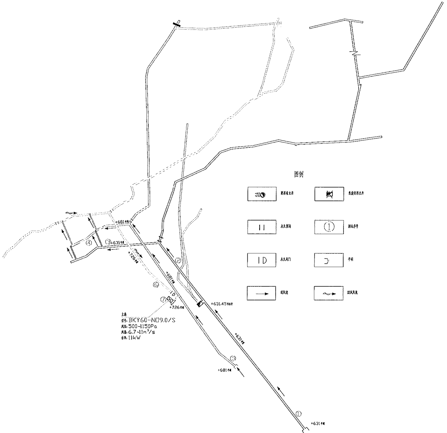
江西华源矿业科技有限公司大王尖萤石矿通风系统测点布置示意图
