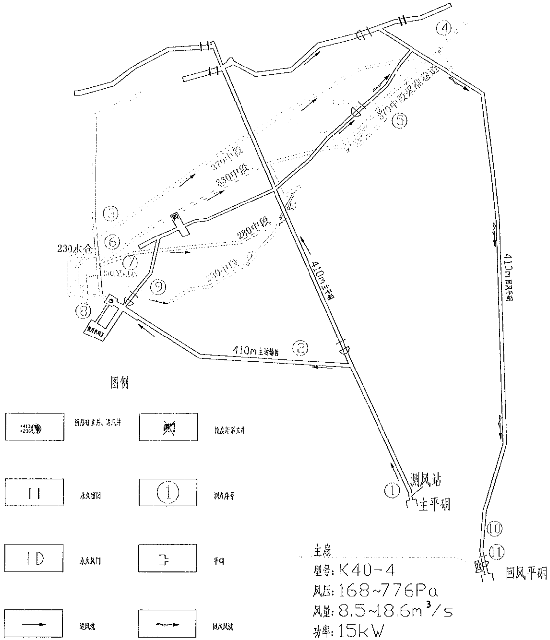
横峰县葛源金星萤石矿通风系统测点布置示意图
