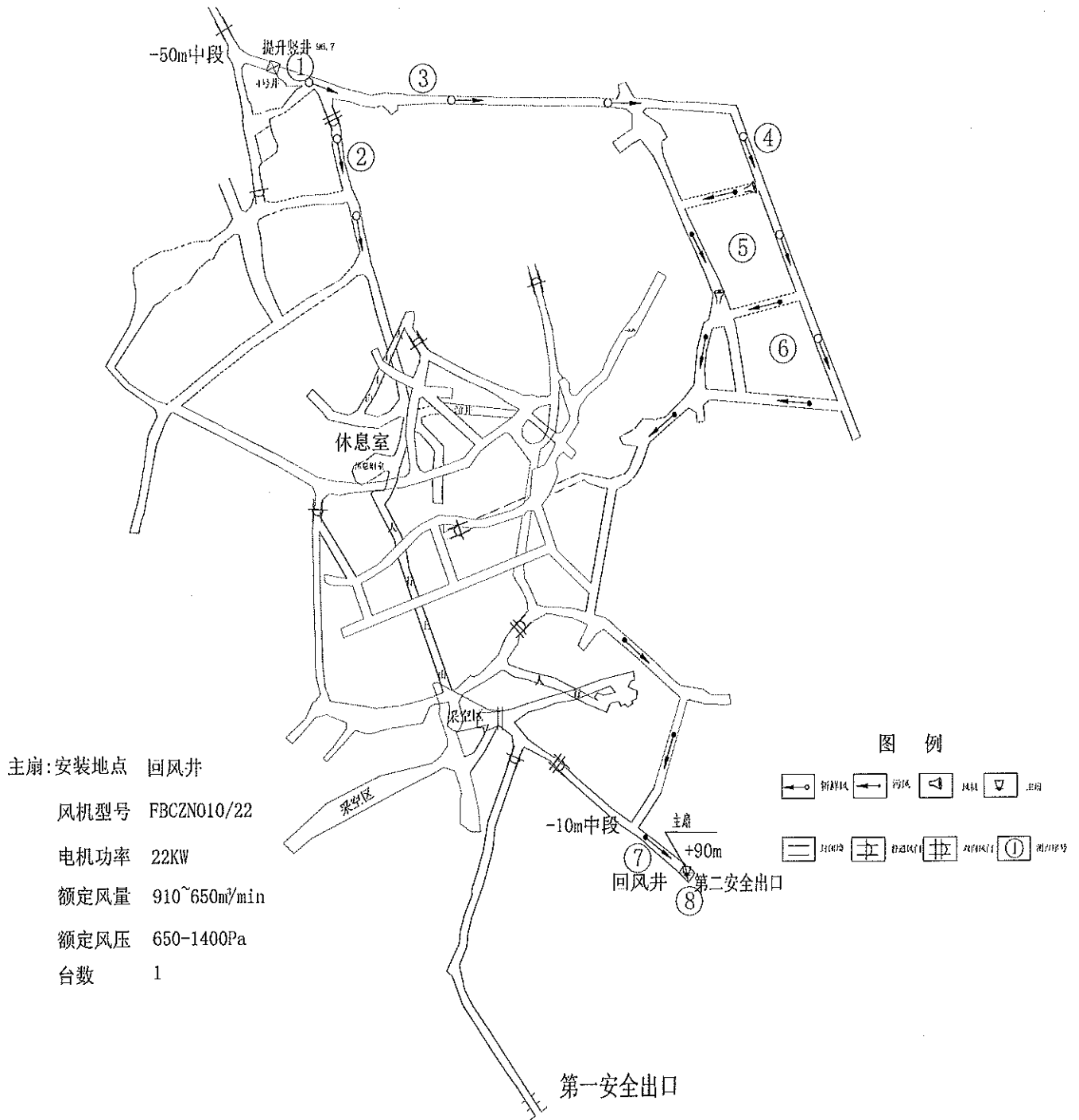
江西省德兴市渔塘金矿通风系统测点布置示意图
