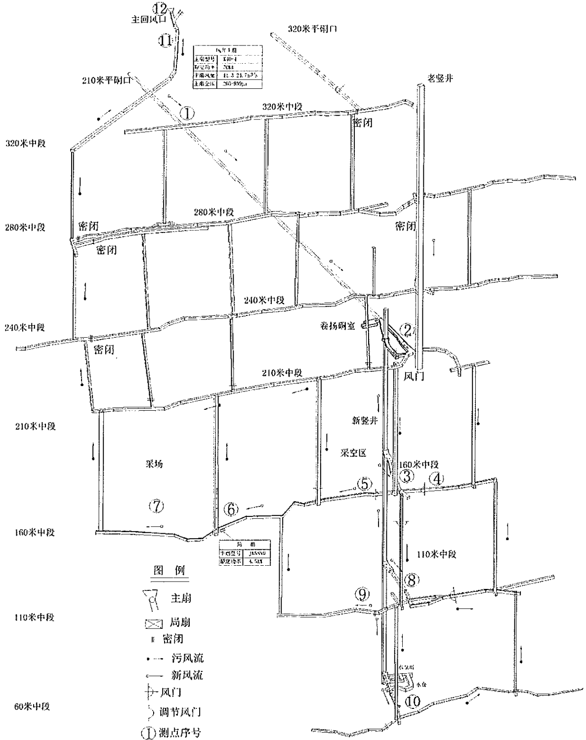
铅山县蓝翔矿业有限公司蓝翔铅锌矿通风系统测点布置示意图
